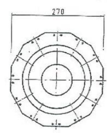
umlaufende Störkontur
