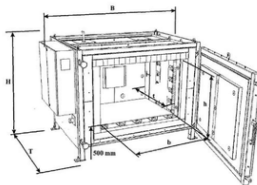
Abb. 5: Abmessungen (Abbildung ähnlich)
